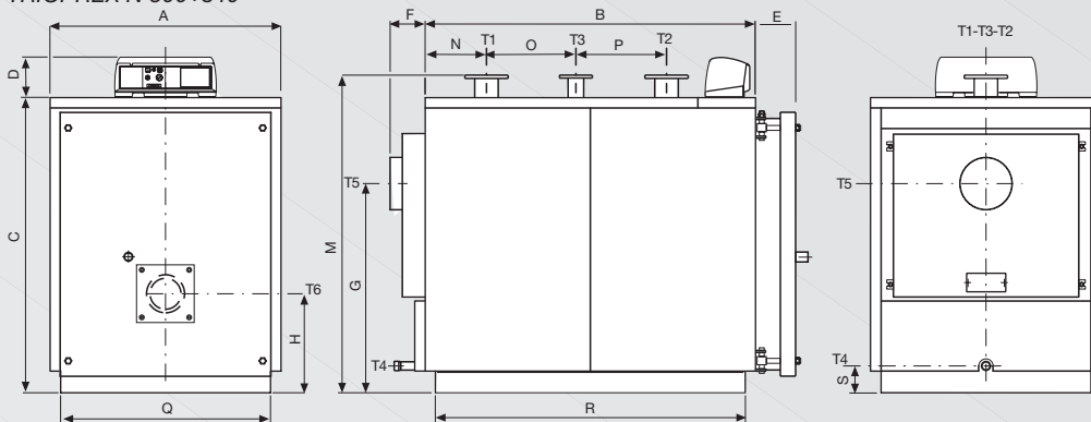
TRIOPREX N 1100÷1900
