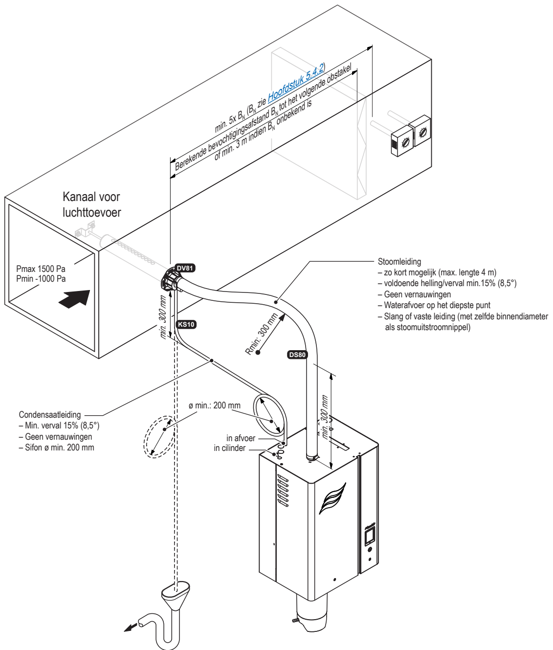
Afb. 14: Overzicht stoominstallatie kanaalbevochtiging
