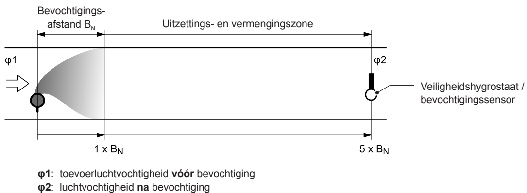
Afb. 16: Bevochtigingsafstand " B_N "
