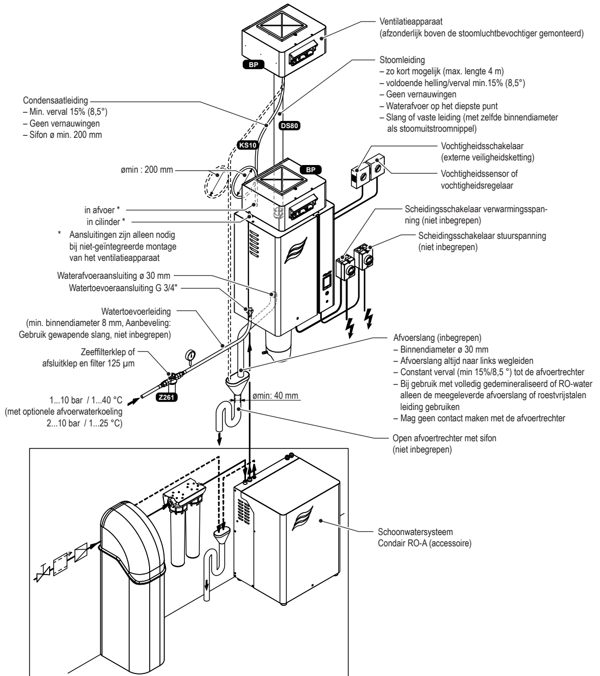
Afb. 8: Typische installatie voor directe ruimtebevochtiging
