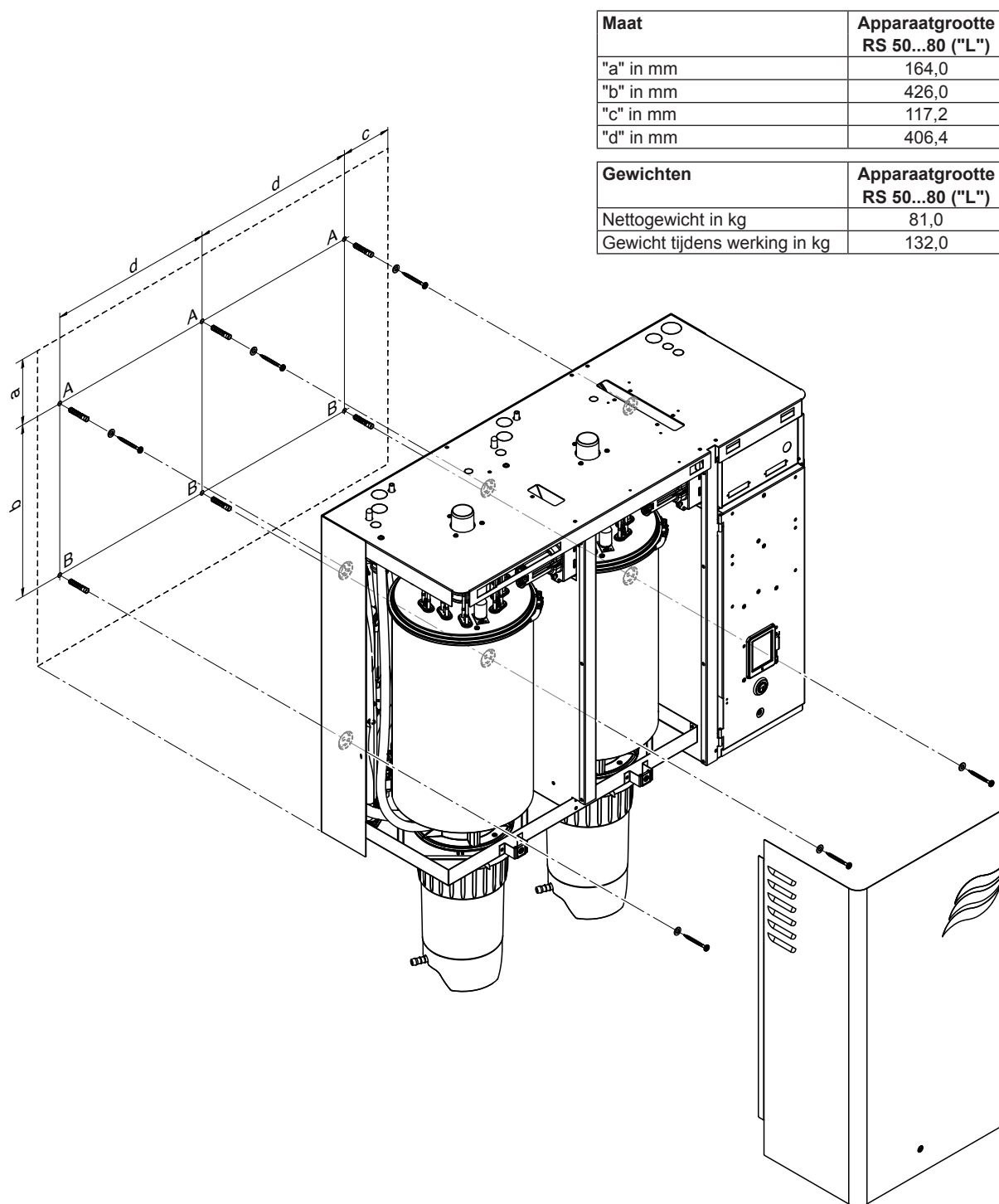
Afb. 11: Overzicht standaardmontage stand-aloneapparaten groot formaat
