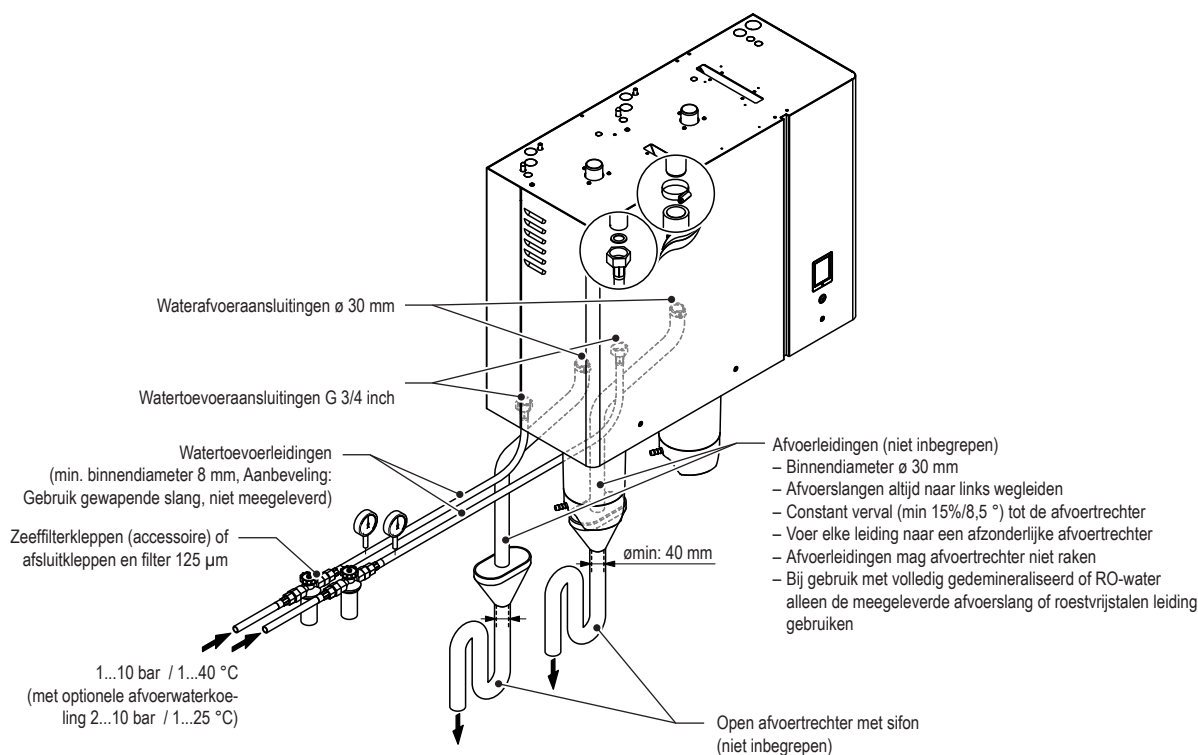
Afb. 22: Overzicht waterinstallatie voor stand-aloneapparaten groot formaat
