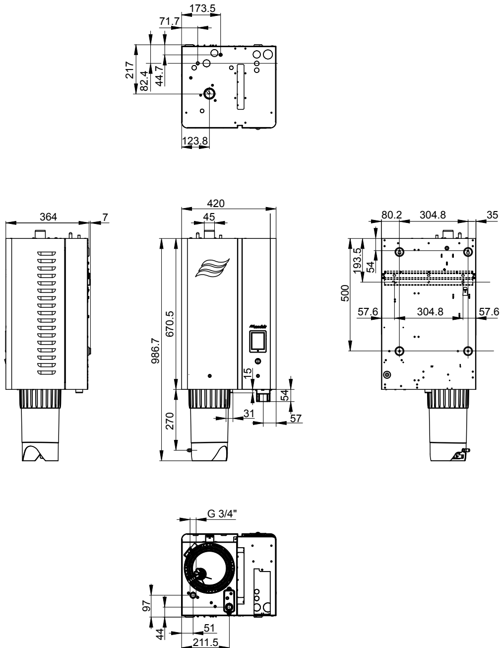
Afb. 31: Maattekening apparaat "S" (afmetingen in mm)
