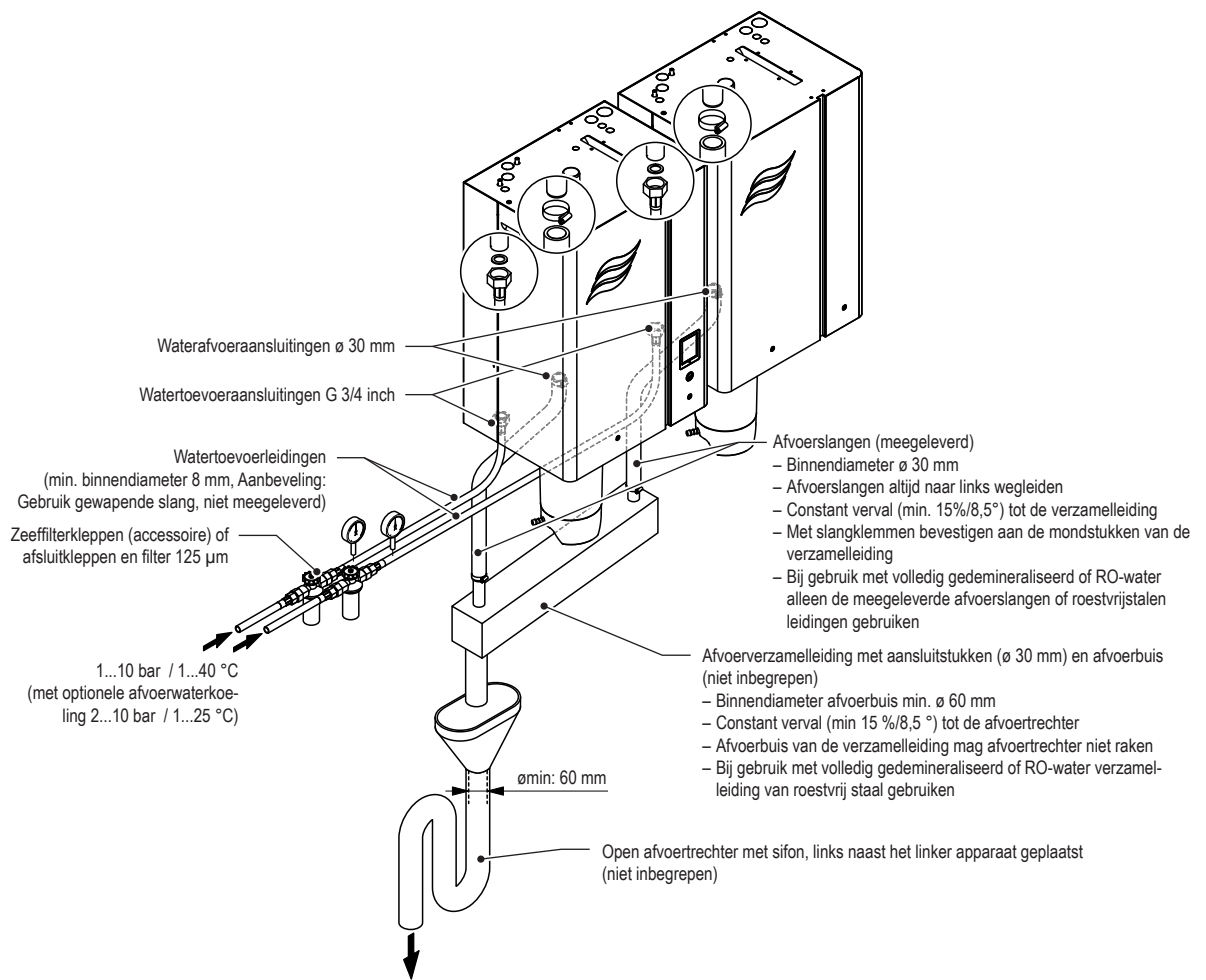
Afb. 23: Overzicht waterinstallatie voor dubbele apparaten middelgroot ("M") formaat
