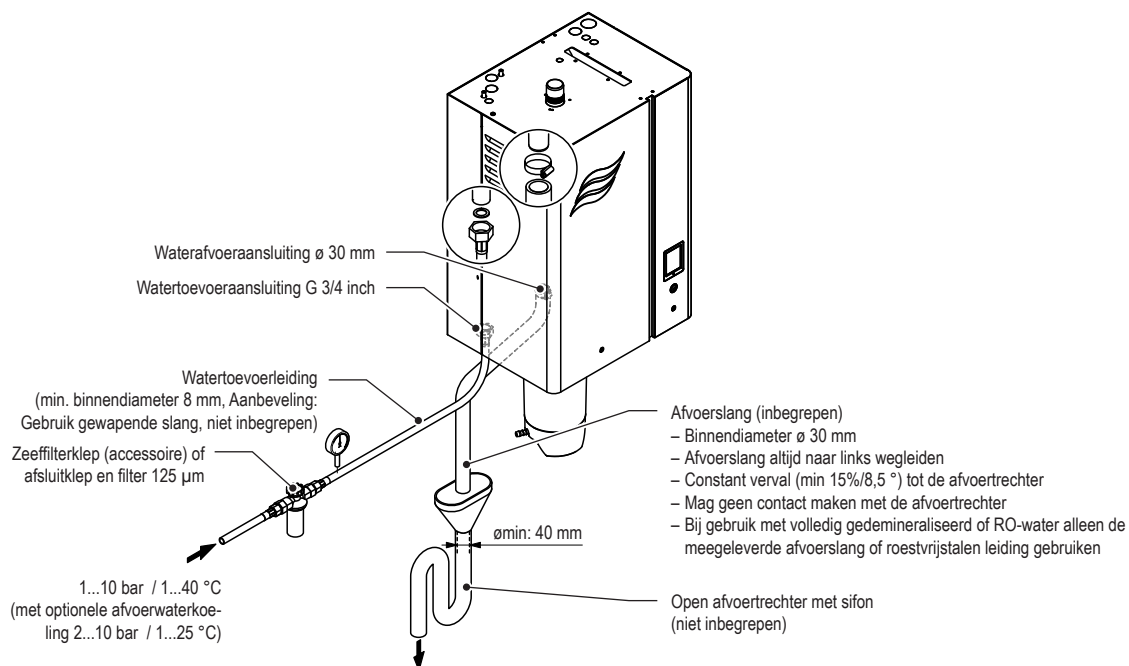
Afb. 21: Overzicht waterinstallatie voor stand-aloneapparaten klein en middelgroot formaat
