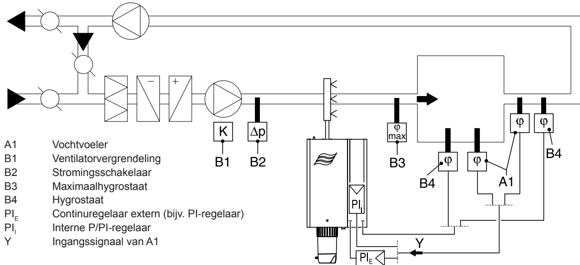
Afb. 24: Systeem 1 – ruimtebevochtigingsregeling
