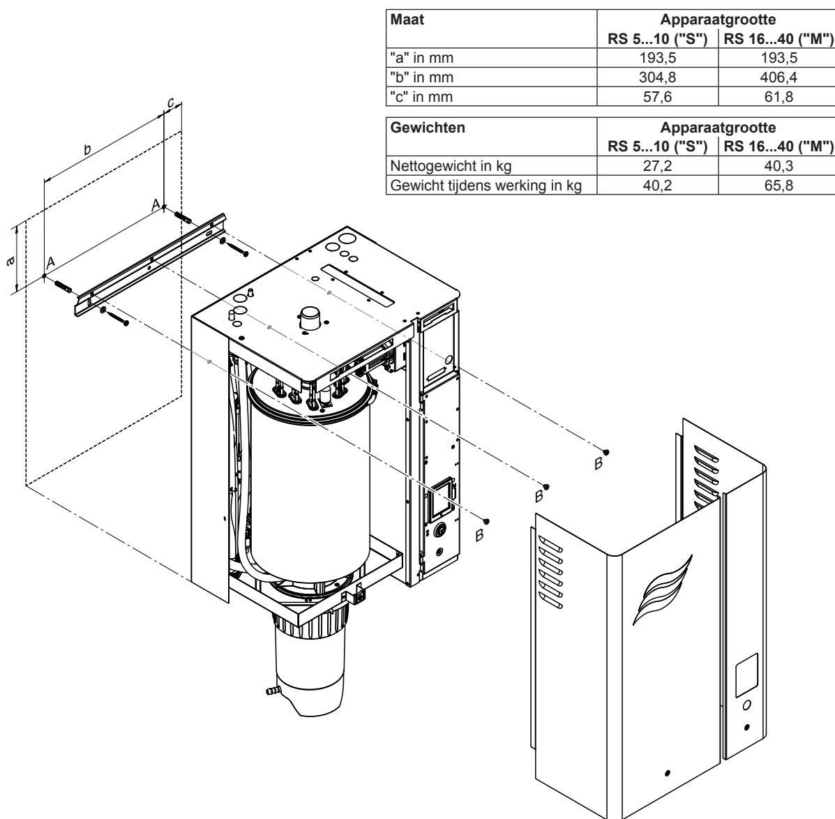
Afb. 12: Overzicht montage van stand-aloneapparaten klein en middelgroot formaat met wandrek
