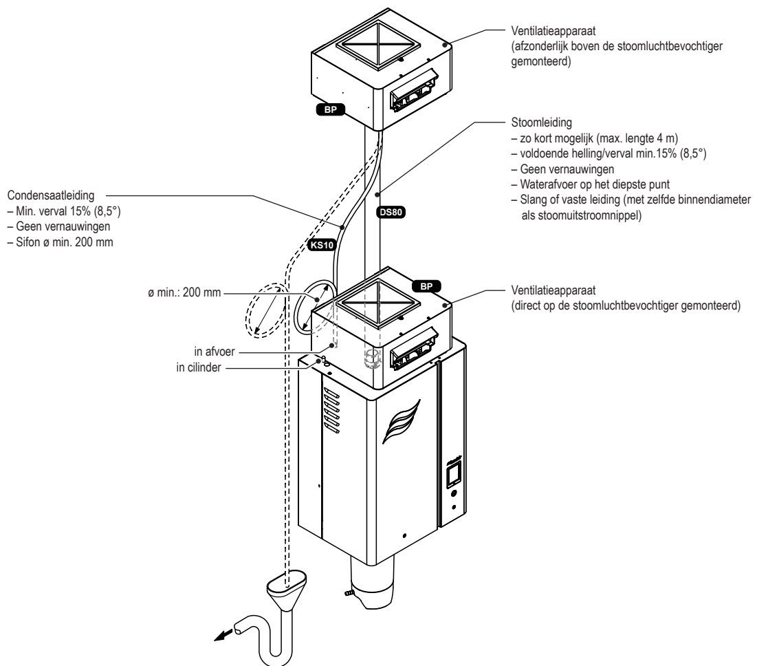
Afb. 15: Overzicht stoominstallatie ruimteluchtbevochtiging
