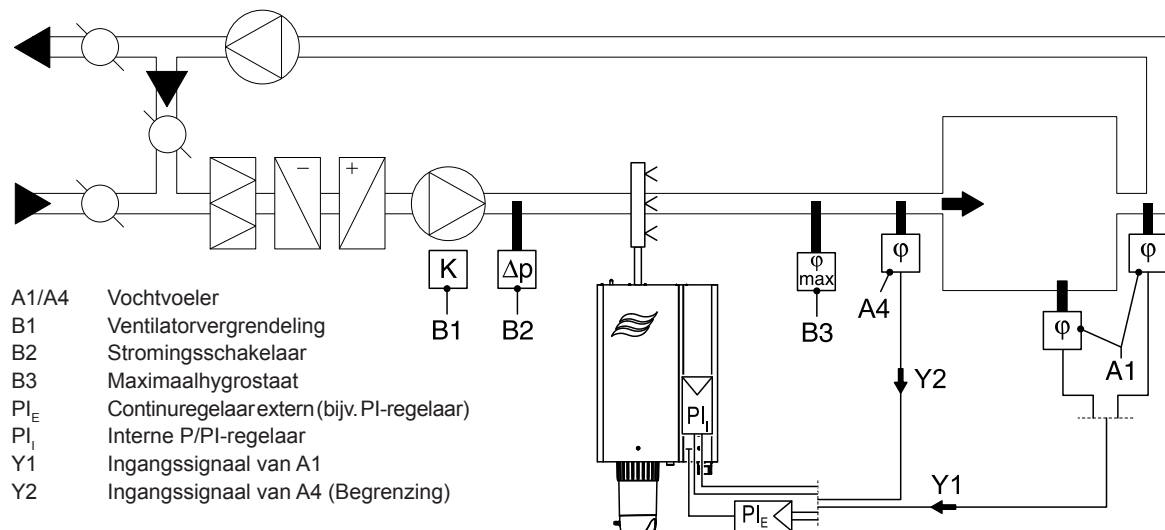
Afb. 25: Systeem 2 – ruimtebevochtigingsregeling met continue begrenzing van het vochtgehalte in de toegevoerde lucht
