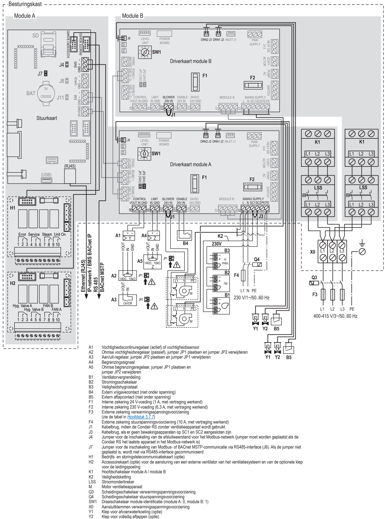
Afb. 28: Elektrisch schema Condair RS 50...80 - stand-aloneapparaten "L"
