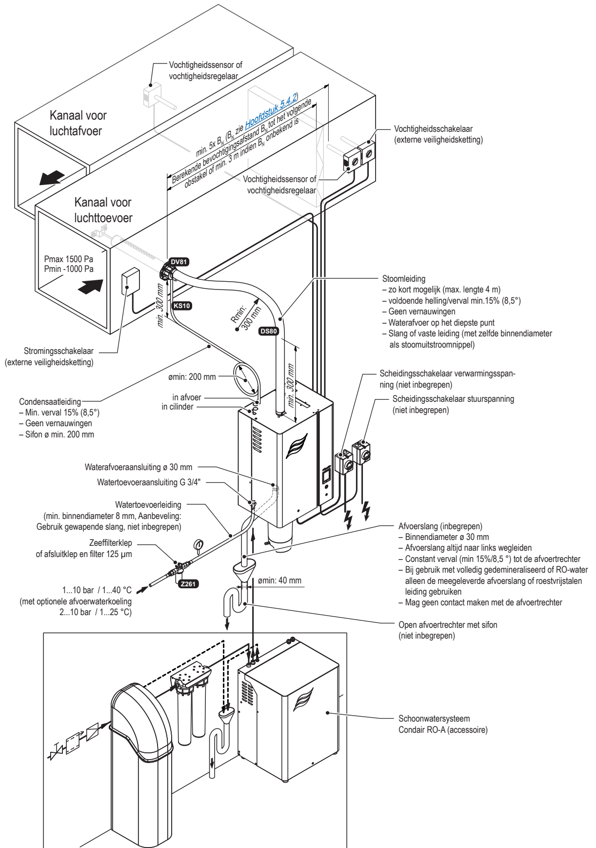
Afb. 7: Typische installatie voor kanaalbevochtiging
