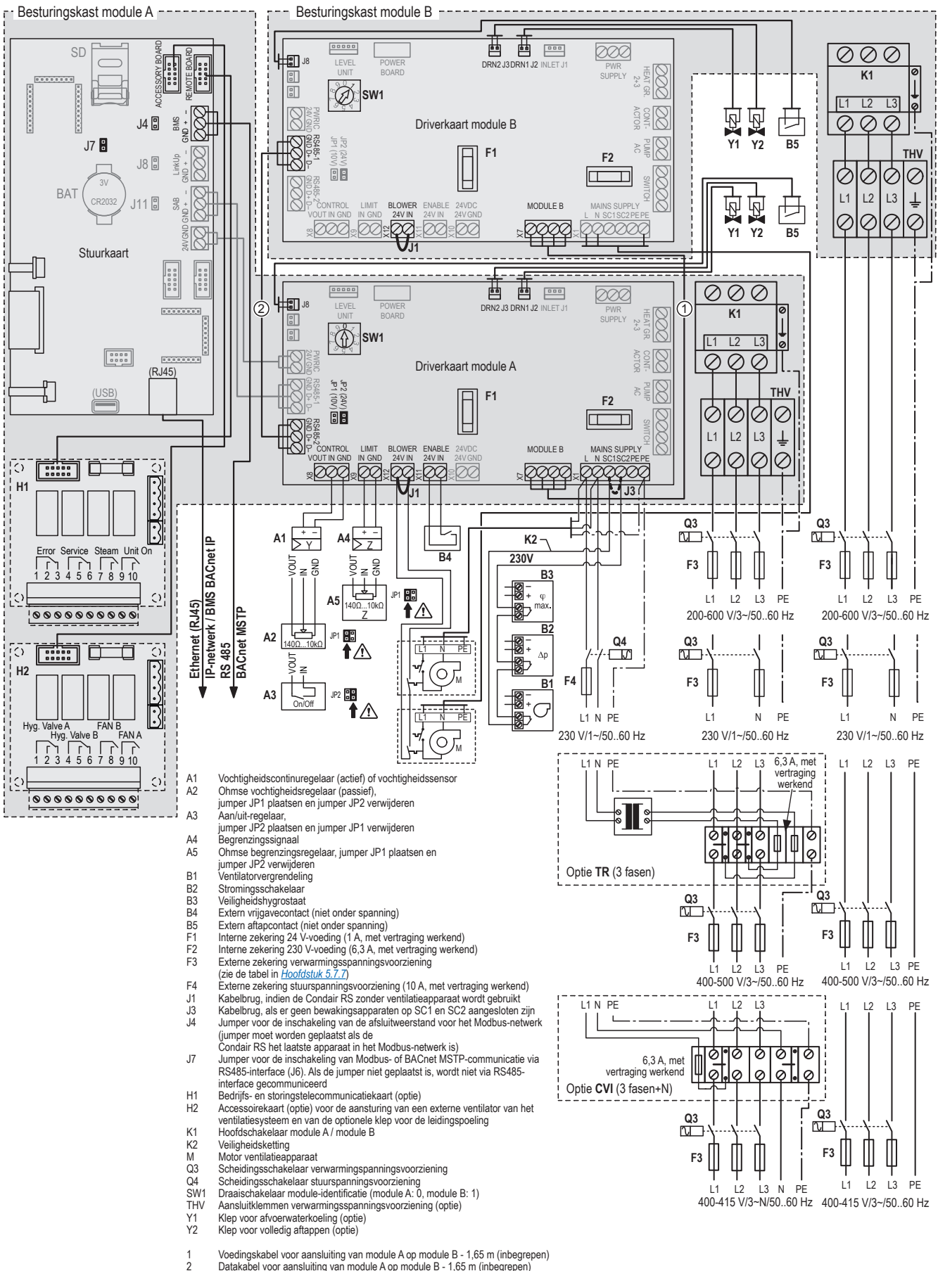
Afb. 29: Elektrisch schema Condair RS 40...80 - dubbele apparaten 2x "M"
