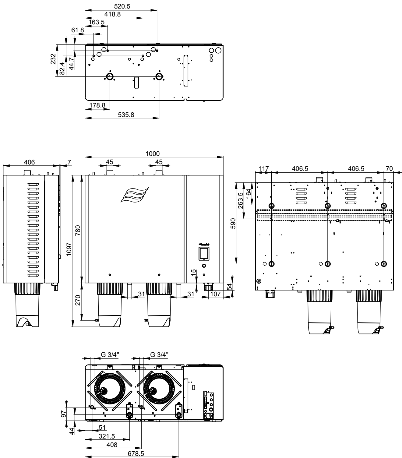
Afb. 33: Maattekening apparaat "L" (afmetingen in mm)
